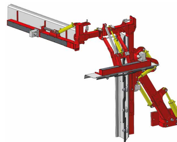
VERSIONE CON PISTONE PER RETRAIBILITÀ BARRA VERTICALE PIÙ ESTERNA (0-90°) + MOLLA DI SICUREZZA ANTIURTO.
