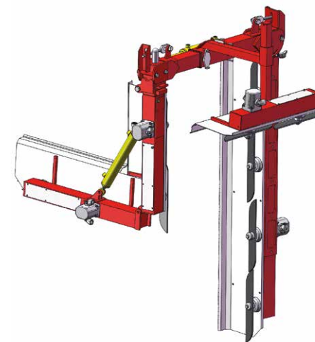
VERSIONE CON ULTIMI DUE COLTELLI RETRAIBILI (0-90°), SU BARRA VERTICALE PIÙ ESTERNA CON PISTONE IDRAULICO.
