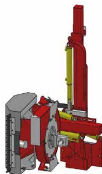
VERSIONE COMPATTA CON PIANTONE INCLINABILE IDRAULICAMENTE
